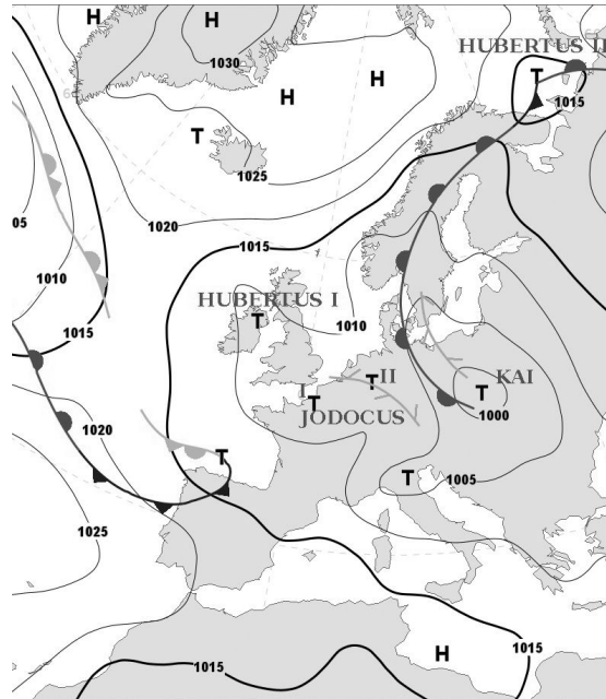
ABB. 28 Die Wetterkarte vom 11. Mai 2021: Tief „Jodocus“ über Mitteleuropa.
